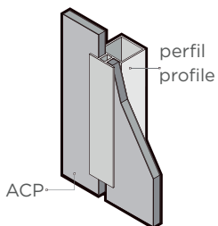
Fijación por inserción Insertion assembly
