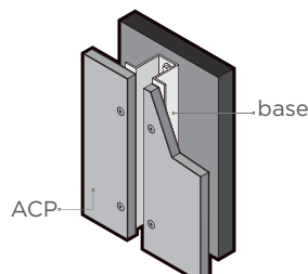
Fijación con remache expuesto Riveted exposed
