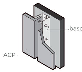
Fijación suspendida suspended
