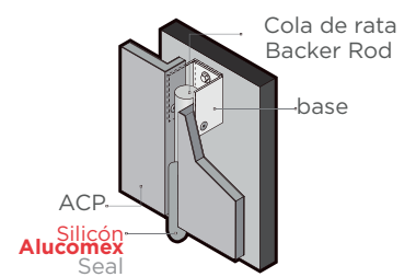
Fijación mecánica Screwed tray
